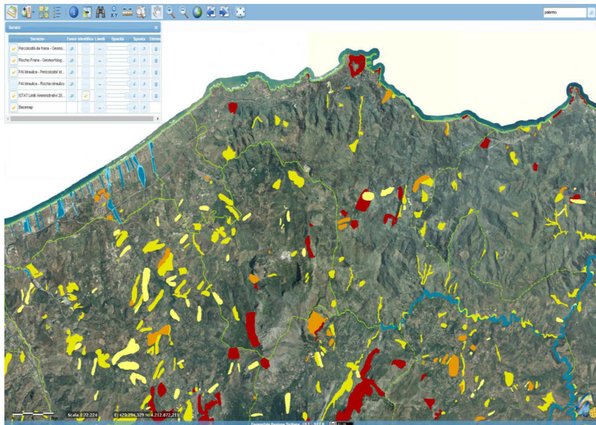
Fig. 7 - Aree di criticità geomorfologiche e idrauliche, dal livello 1 al livello 4, individuate dal Piano per l'Assetto Idrogeologico nel territorio di Cefalù
