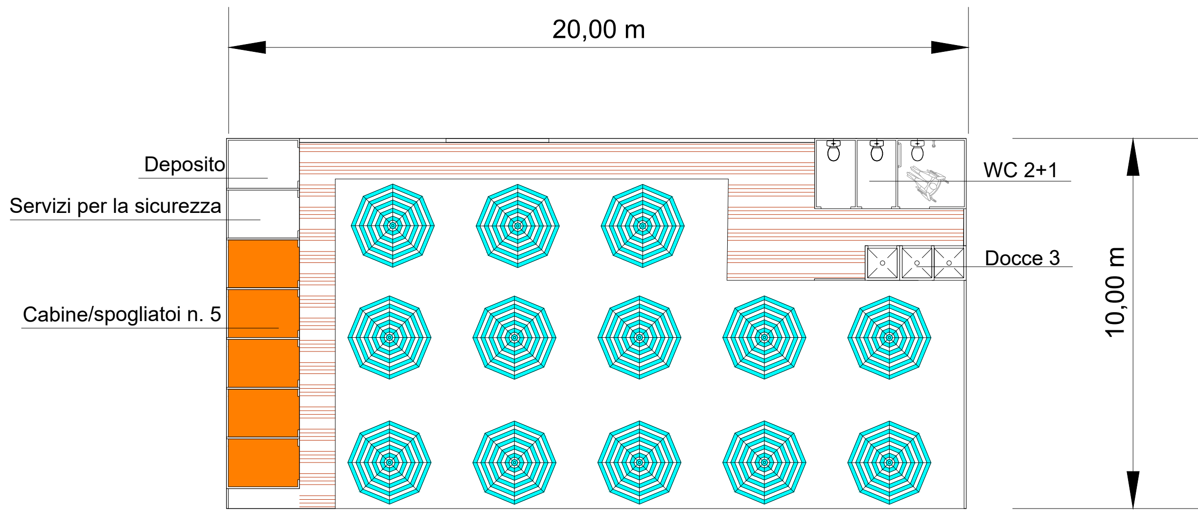
Area attrezzata per la balneazione - Lotto tipo n. 18
