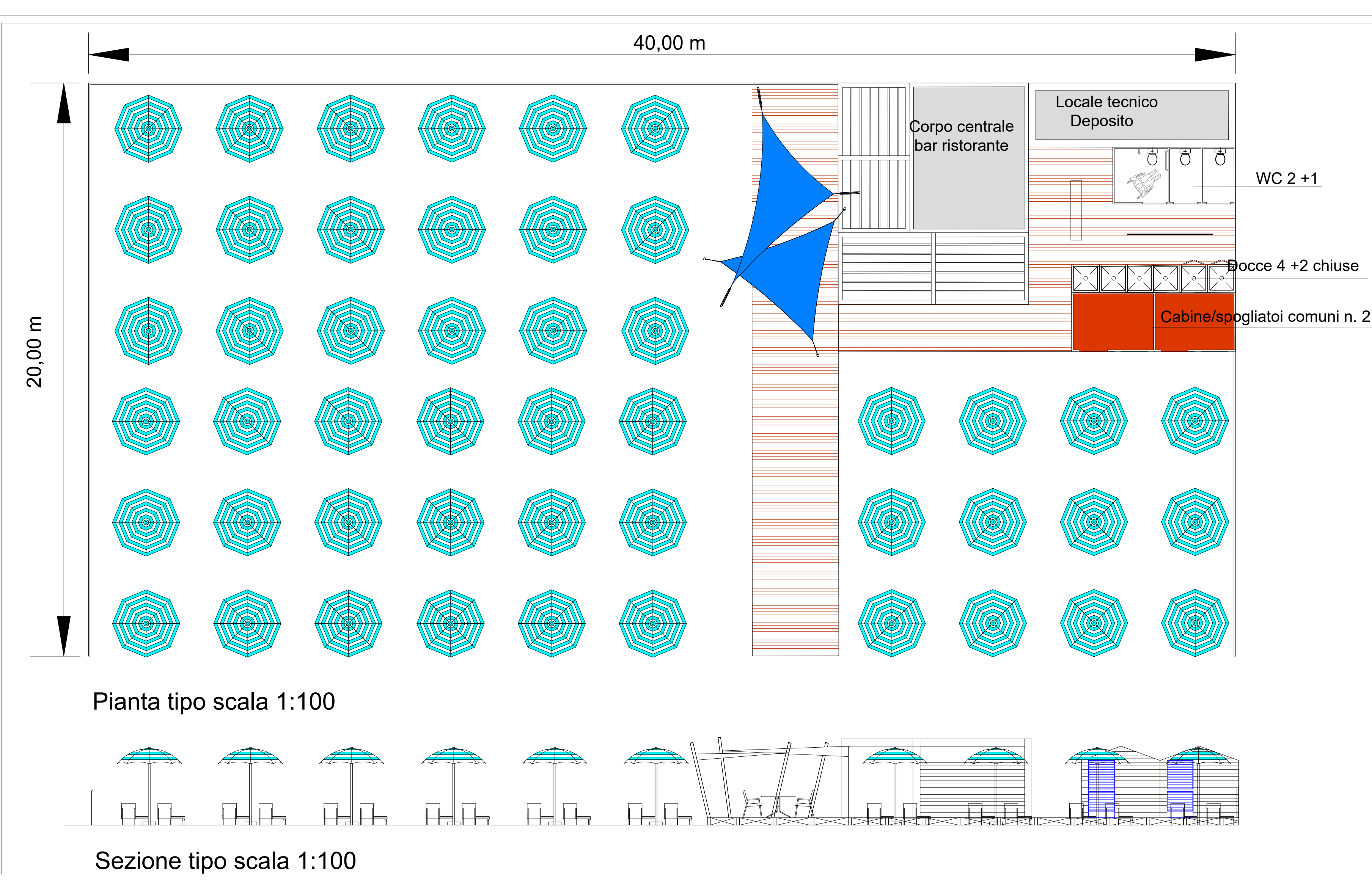
Stabilimento balneare - Lotto tipo n.24
