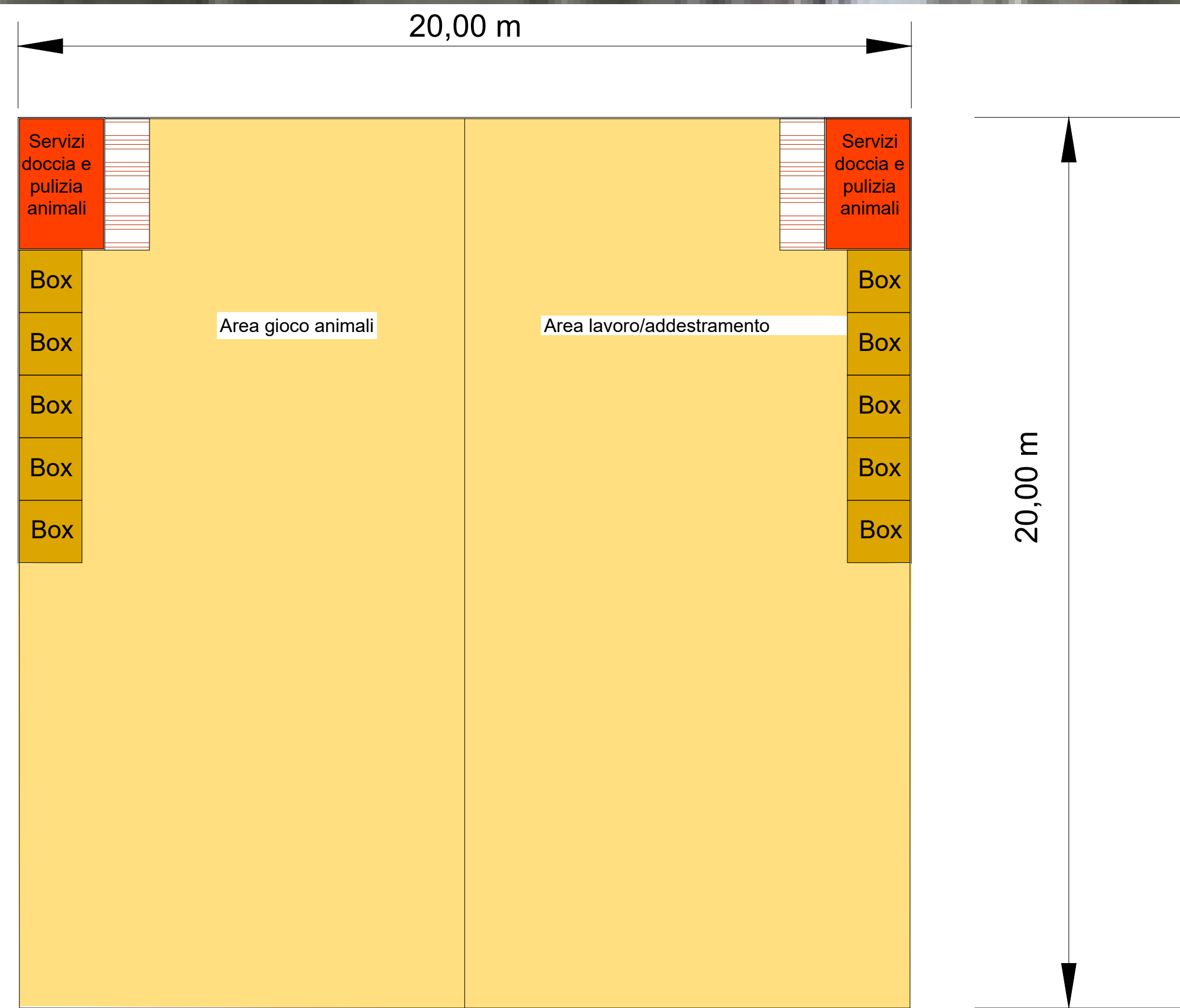
Area per animali di affezione - Lotto tipo n.2
